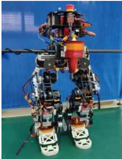
Вид летающего робота-гуманоида Jet-HR2
