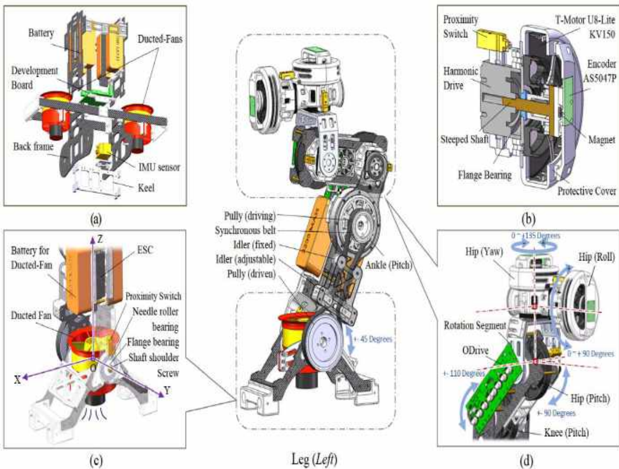
Сборка механических компонентов ноги робота: (а) Талия (b) Модульный сустав, используемый в бедре и колене (c) Ступни (d) Бедро
