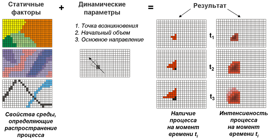
Рис. 5. Расчет целевой функции с помощью «дисперсионных моделей»
