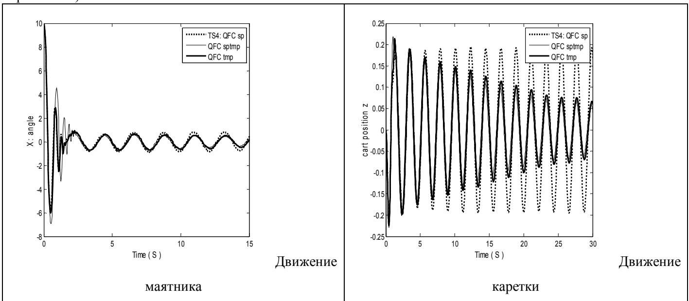
Рис. 22. Динамическое поведение системы «маятник-каретка» при управлении КНВ с тремя типами корреляций
