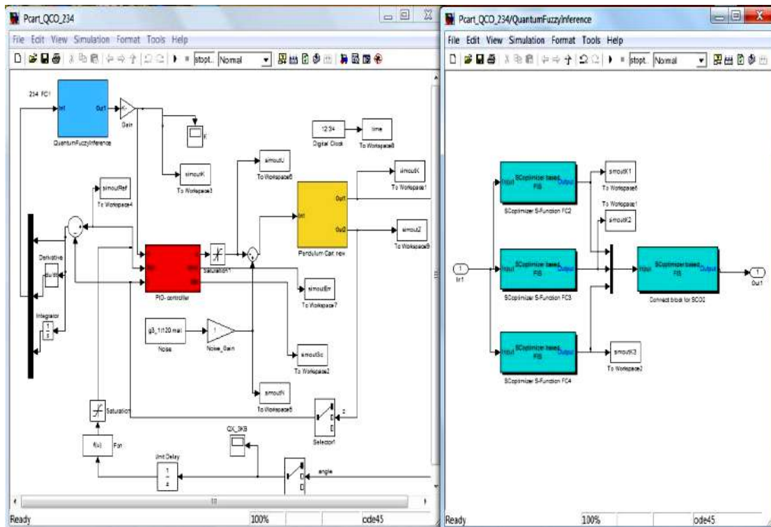
Рис. 20. Матлаб/Симулинк структура квантового регулятора динамической системы «маятник-каретка»
